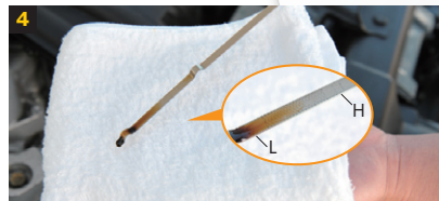
4 もう一度抜いてオイルの量がオイルレベルゲージの規定の範囲内(HとLの間)にあるかを確認します。
